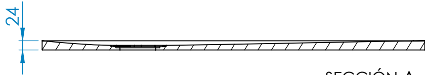
SECCIÓN A-A
