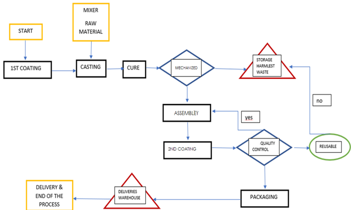
Figura 3: Esquema de flujo simplificado del proceso productivo de las encimeras Akron.
